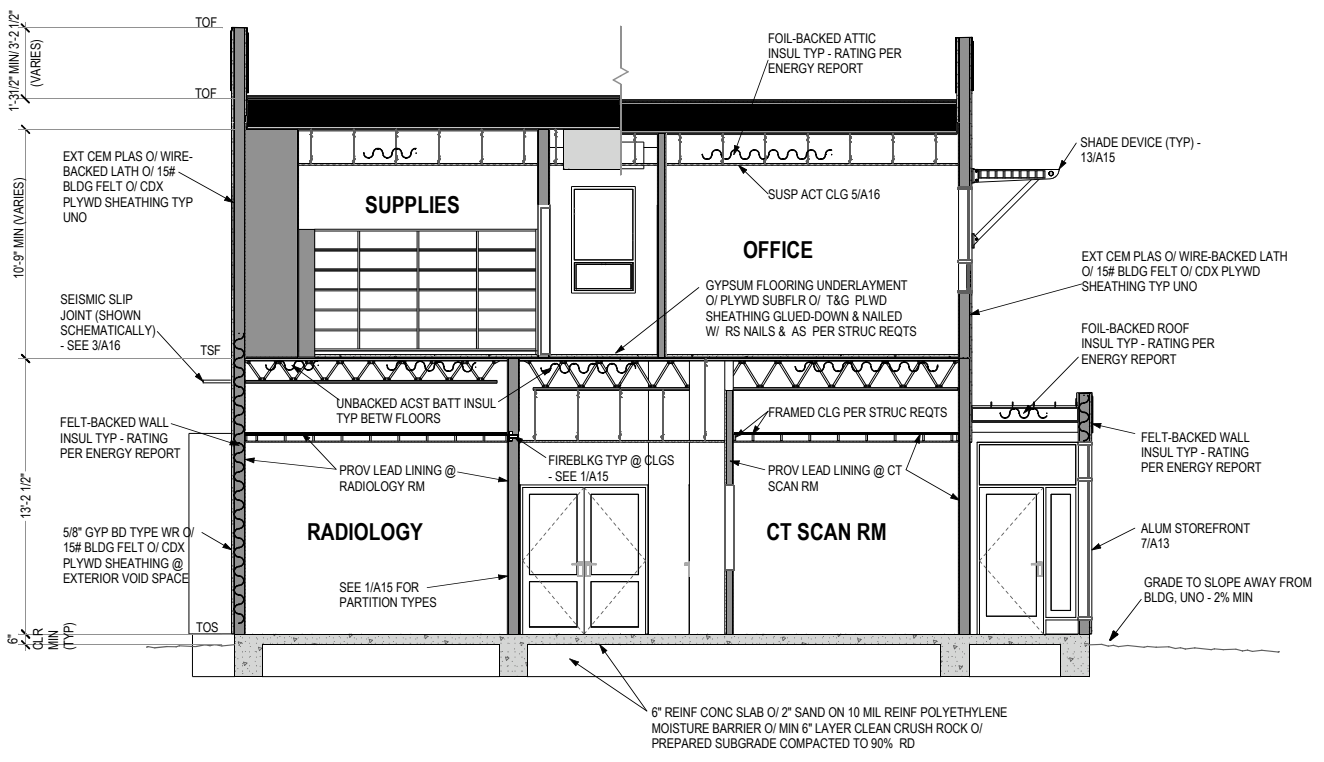
SECTION D - D' 1/4" = 1'-0"
